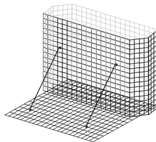
ST – Basiskorb mit Gitterboden und rückwärtigen Zugankern
